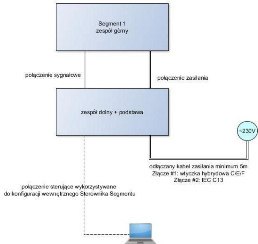
Rysunek 2. Przykład okablowania dla pojedynczego Segmentu
