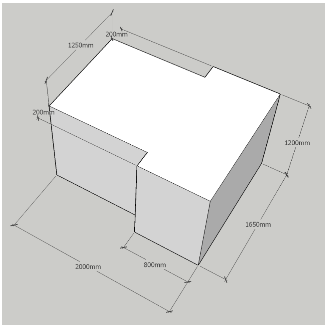
Rysunek 1. Maksymalny gabaryt zajmowany przez komplet skrzyń transportowych zawierających pełną Wideoscianę
