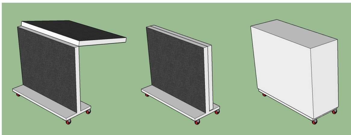
Rysunek 5. Przykładowe rozwiązanie demontażu środkowego zestawu modułów LED oraz umieszczenie Segmentu w skrzyni transportowej.
