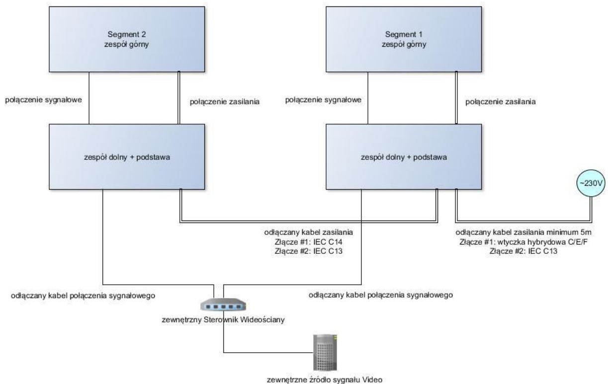
Rysunek 3. Przykład okablowania dla konfiguracji Wideościany złożonej z wielu Segmentów
